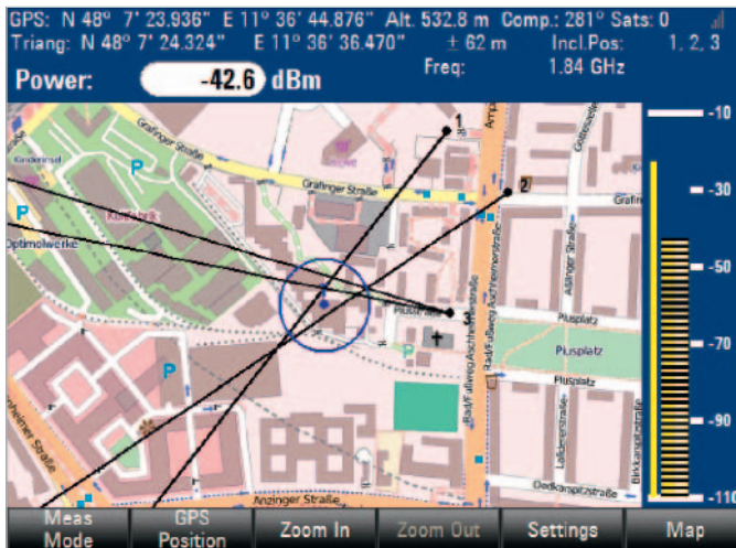
采用R&S®FSH-K15显示地图三角线
