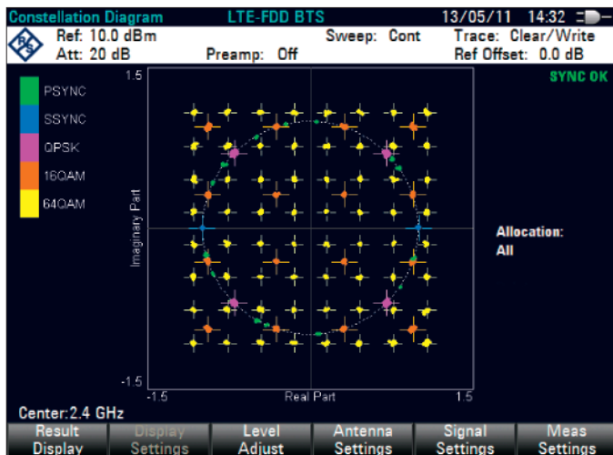
R&S®FSH-K50E选件的星座图以图形方式概述LTE发射信号质量
