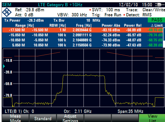
对LTE信号进行频谱发射模板测量
