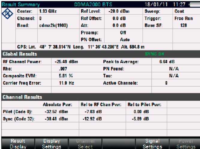
运用R&S®FSH-K46选件分析CDMA2000®发射信号
