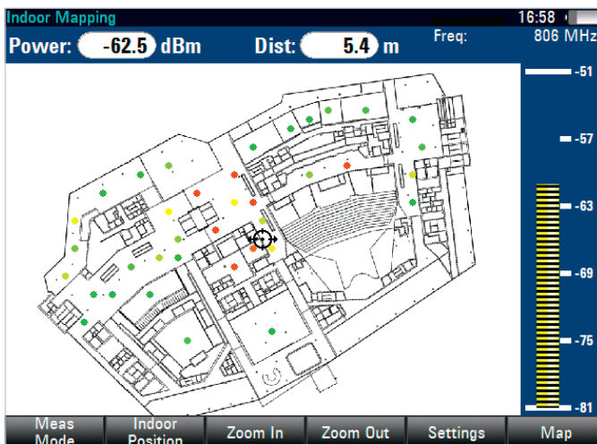
采用R&S®FSH-K17显示室内图
