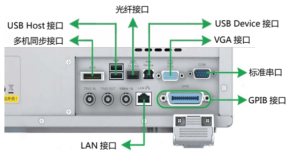
PA8000、PA5000H、PA6000H接口图
