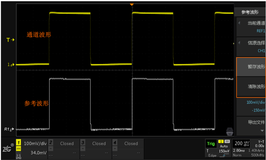
图 21.5 参考波形显示与对比
