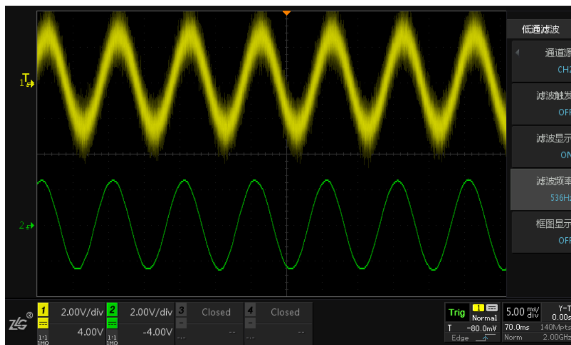
图 17.6 噪声滤波效果图
