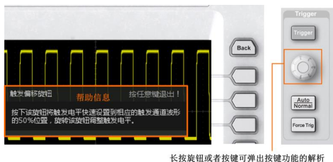
图 5.25 按键帮助信息
