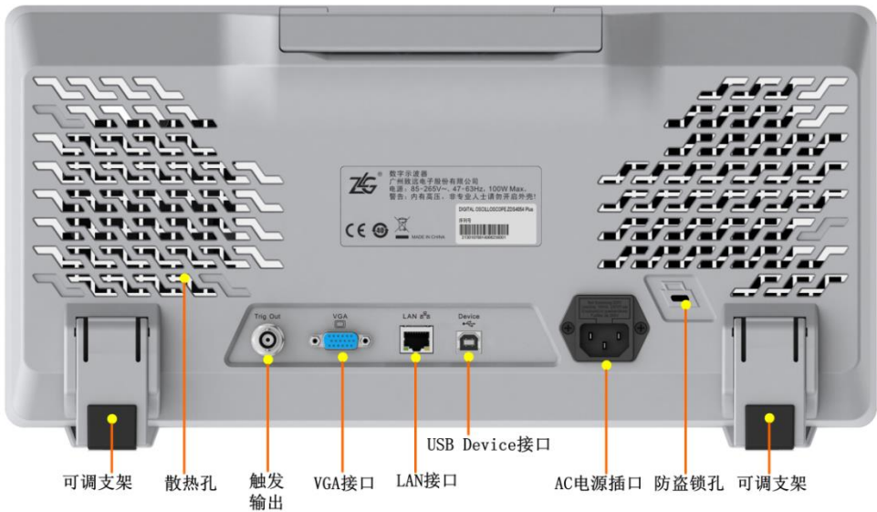
图 5.9 ZDS4054 Plus 型示波器后面板
