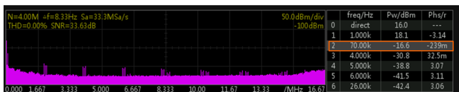
图 19.10 FFT 频谱表操作
