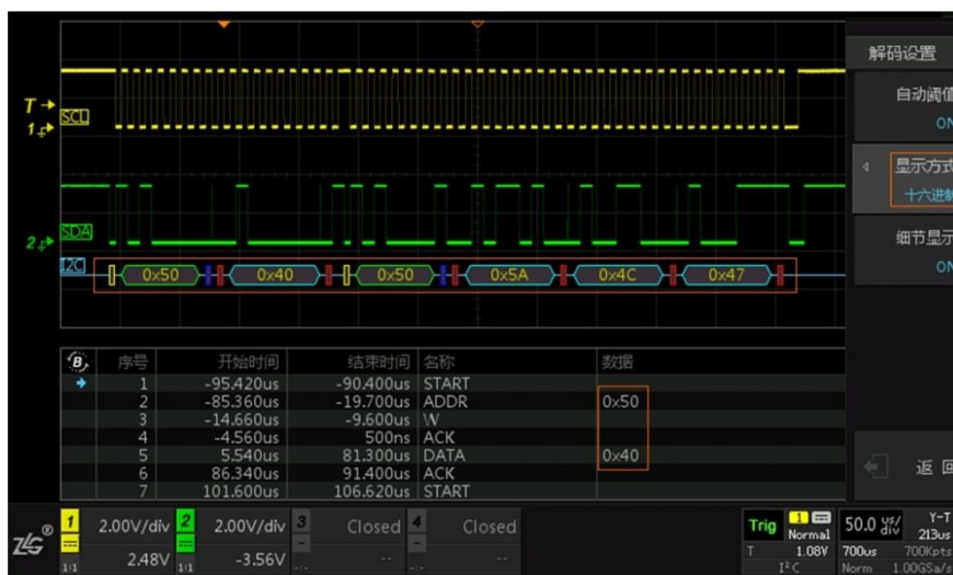
图 15.27 十六进制显示
