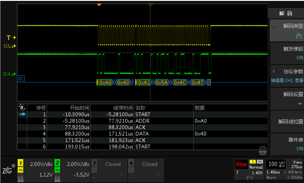
图 15.25 I 2 C 协议解码图（7 位地址模式）
