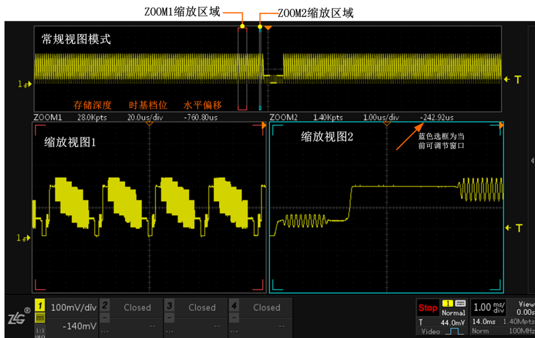
图 6.6 双 ZOOM 显示模式
