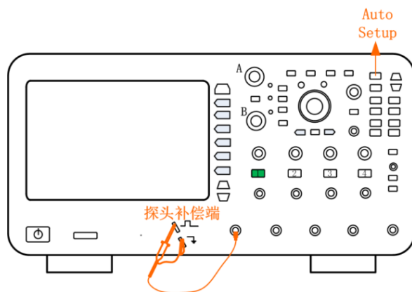
图 5.21 探头接线图
