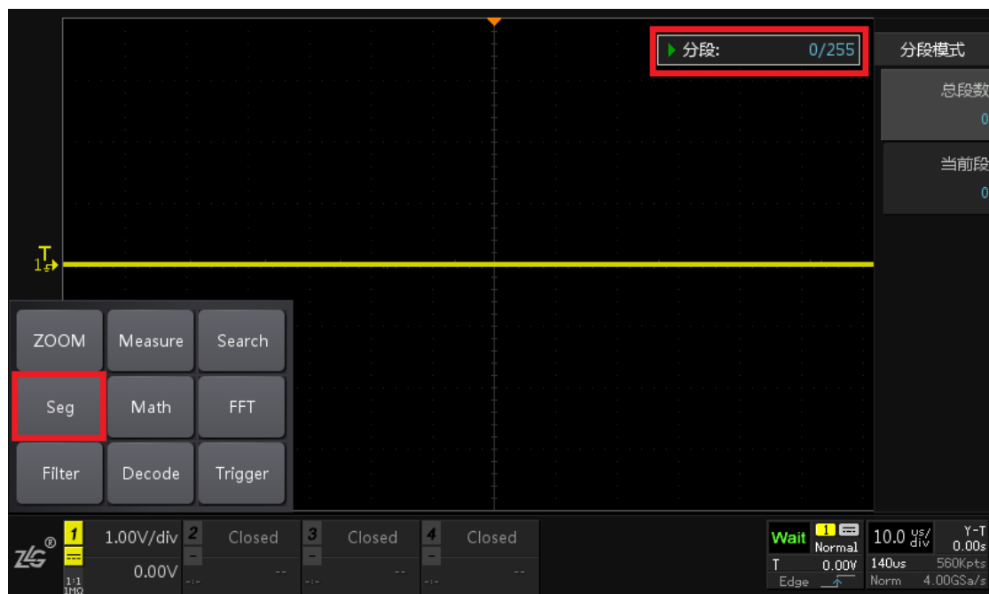
图 20.2 分段存储设置
