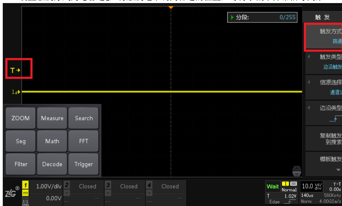
图 20.3 触发方式设置
