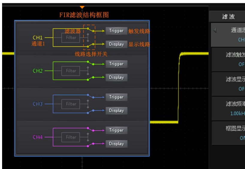
图 17.1 FIR 滤波界面
