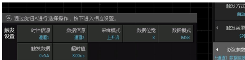
图 10.58 SPI 触发协议参数
