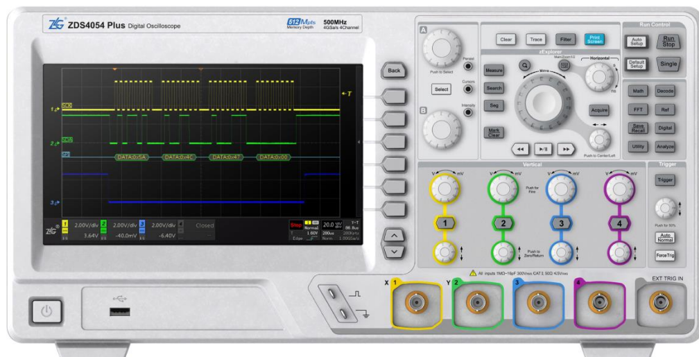
图 3.1 ZDS4054 Plus 示波器面板
