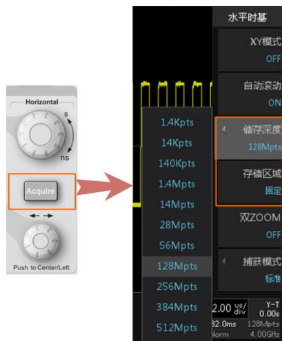
图 6.2 存储深度配置
