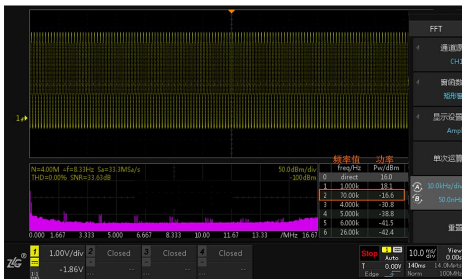
图 19.9 FFT 分析结果
