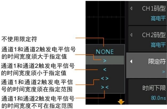
图 10.49 限定符设置说明
