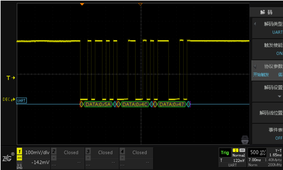
图 15.36 ZDS3000/4000 系列示波器的 UART 信号
