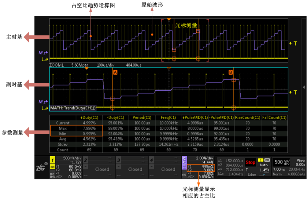
图 18.12 趋势运算界面
