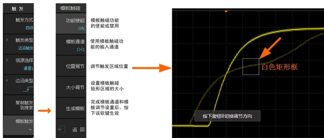
图 10.11 模板触碰功能菜单
