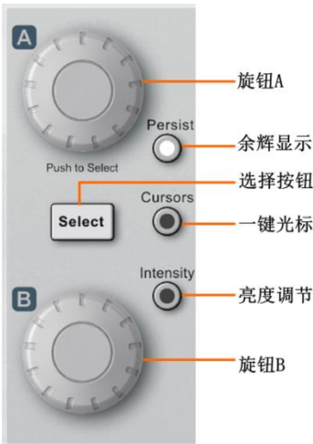
图 5.11 多功能旋钮区面板
