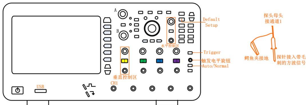
图 13.6 接入毛刺信号
