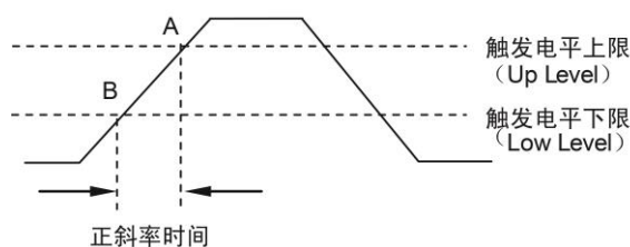
图 10.26 正斜率时间说明
