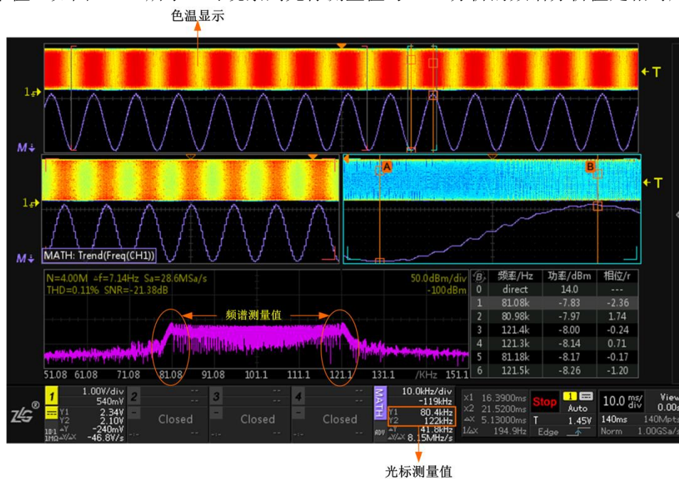
图 18.19 趋势分析效果图
