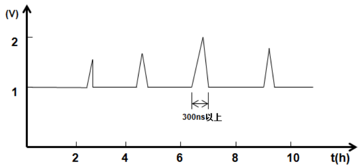
图 20.5 测试波形
