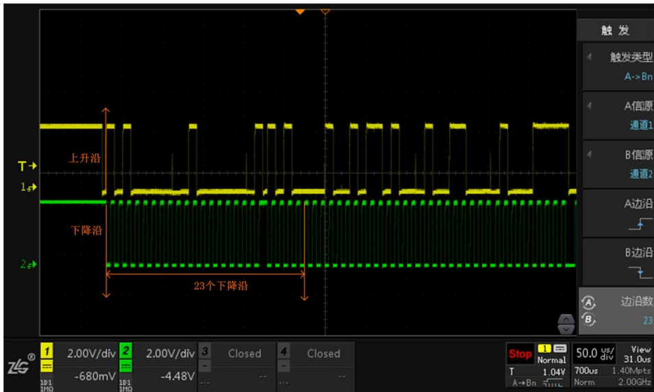
图 10.53 A->B 触发效果图
