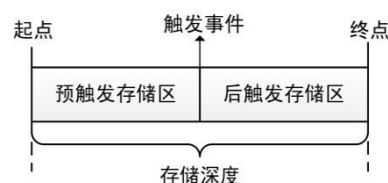
图 6.1 存储深度和可观察区间
