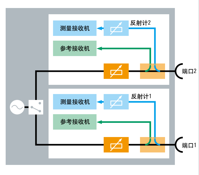
R&S®ZNB双端口型分析仪框图
