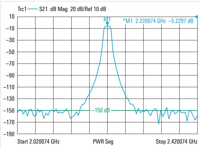
采用分段扫描测量滤波器。
