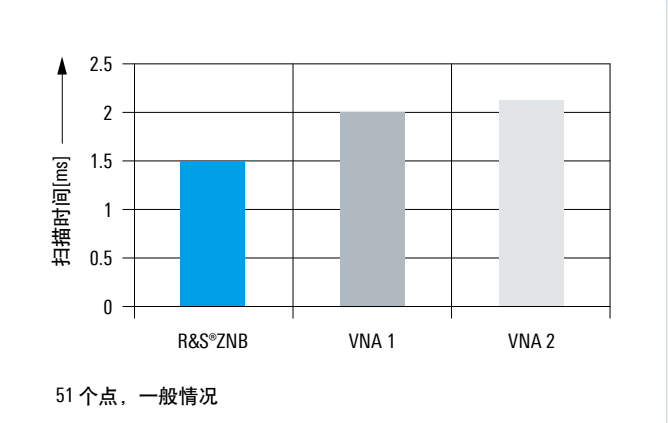
R&S®ZNB与其同类产品的测量速度比较
